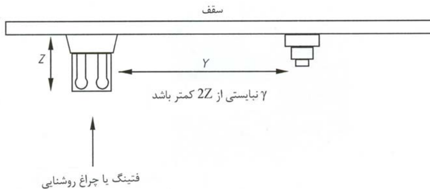
شکل ۴-۸: فاصله آشکارسازها از فیتینگ‌های سقف
