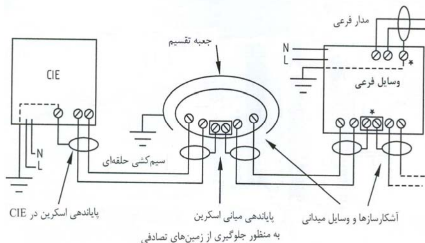
شکل ۴-۱۵ الف : مثالی از سیم‌کشی حلقه‌ای سیستم
