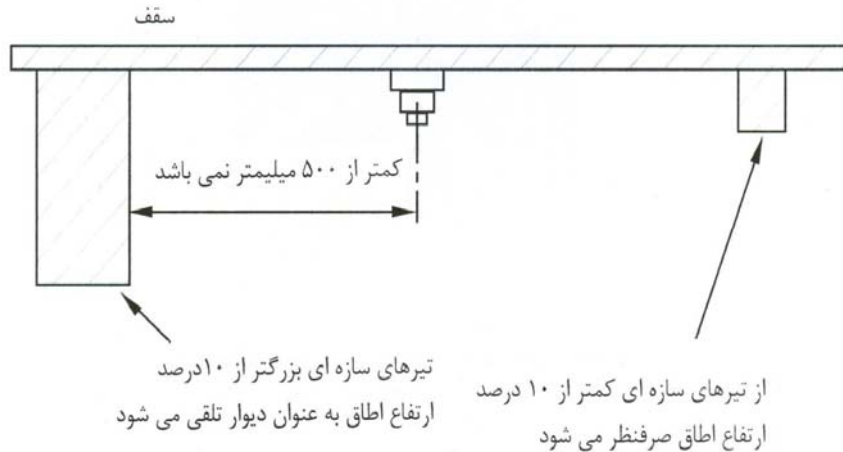
شکل ۴-۱۰ الف : موانع سقفی که دیوار تلقی می‌شوند
