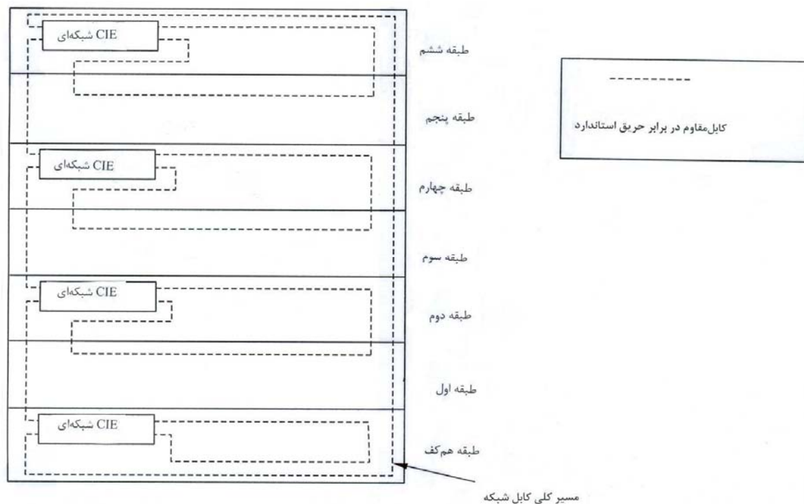
شکل ۴-۱۴ ب: مثالی از سیستم اعلام حریق شبکه‌ای در ساختمان چند طبقه و کاربرد کابل استاندارد در شرایطی که مسيردهی متعددی از حلقه کابل شبکه ای وجود دارد
