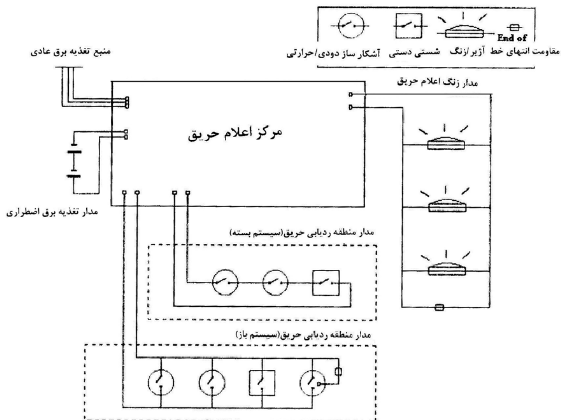
شکل ۱-۲: نمونه سیستم اعلام حریق متعارف
